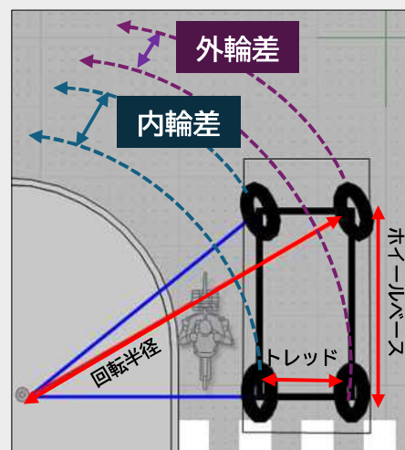
図1. 内輪差・外輪差
